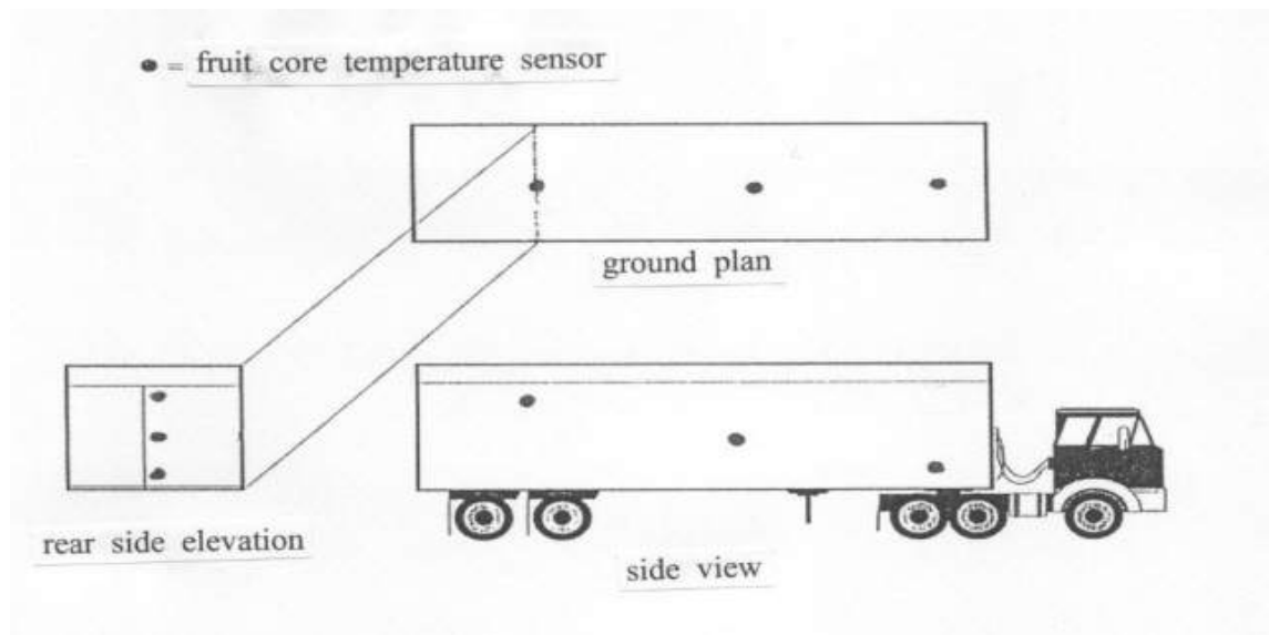
그림. 컨테이너 저온처리 시 과실 중심부 온도센서 설치 위치
